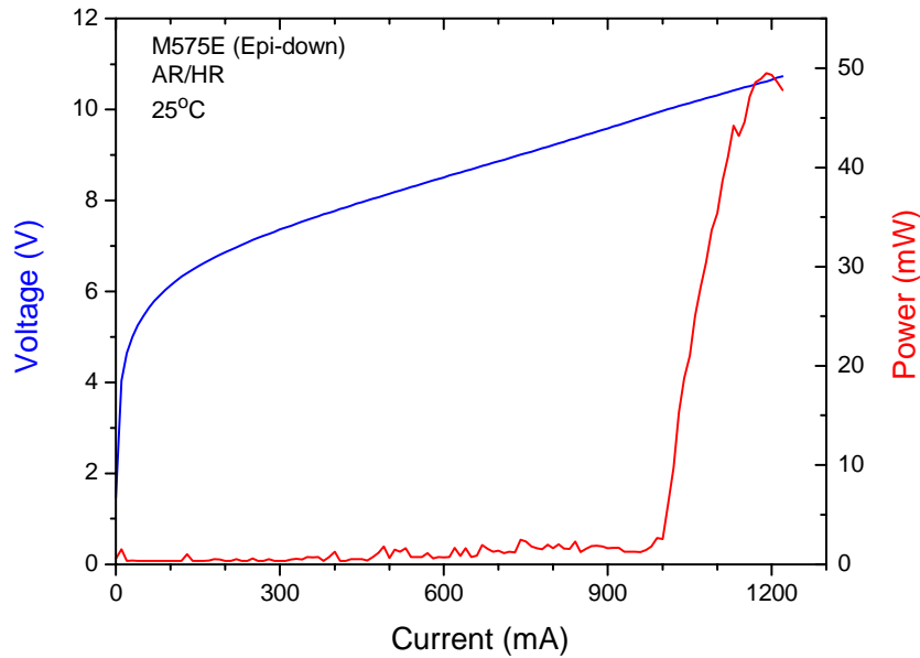
CW L-I-V Characteristics
