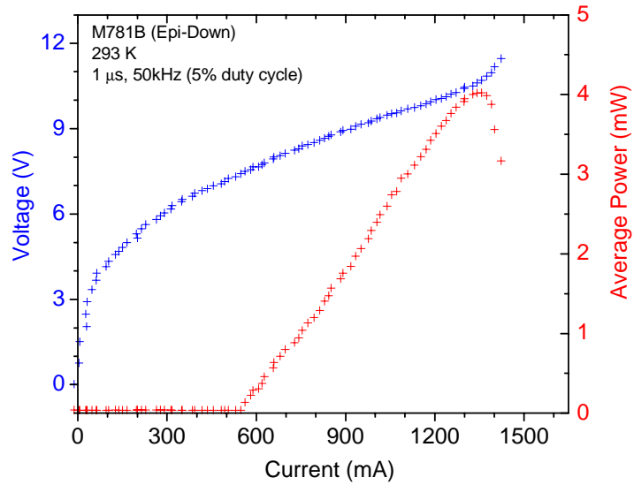
Pulsed L-I-V Characteristics
